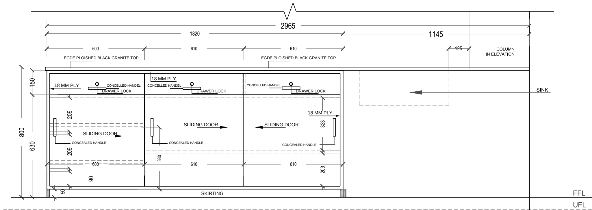
ELEVATION
