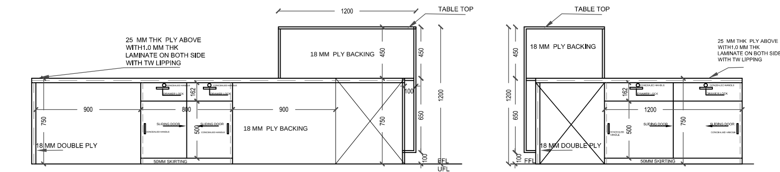
ELEVATION B
