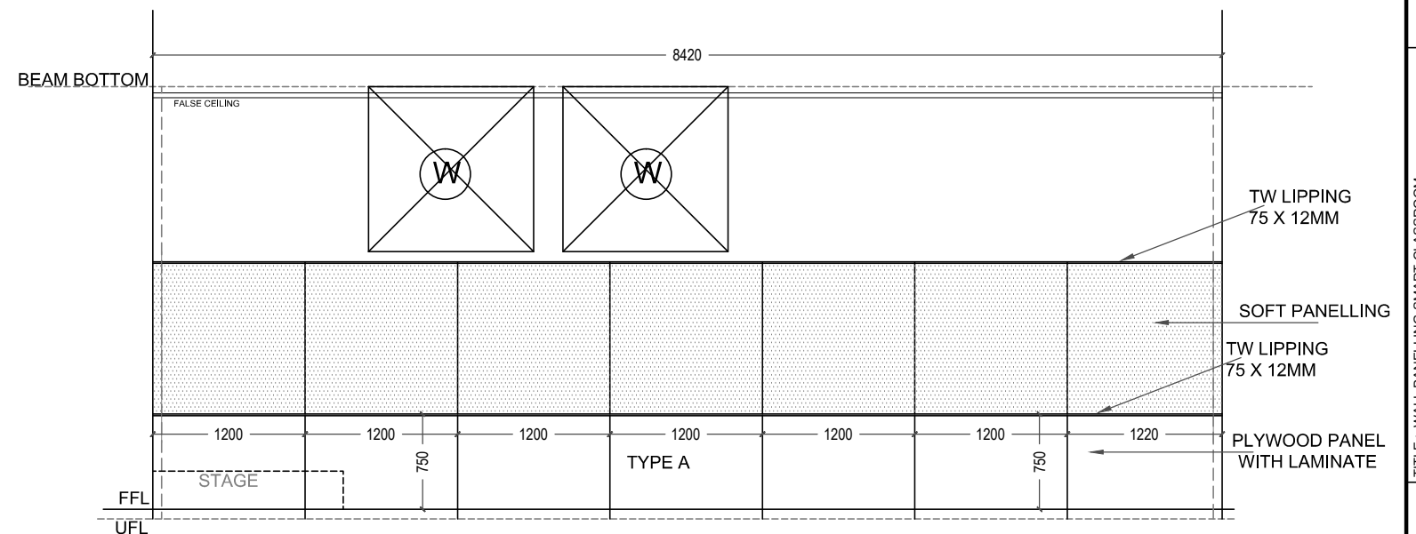
ELEVATION B
