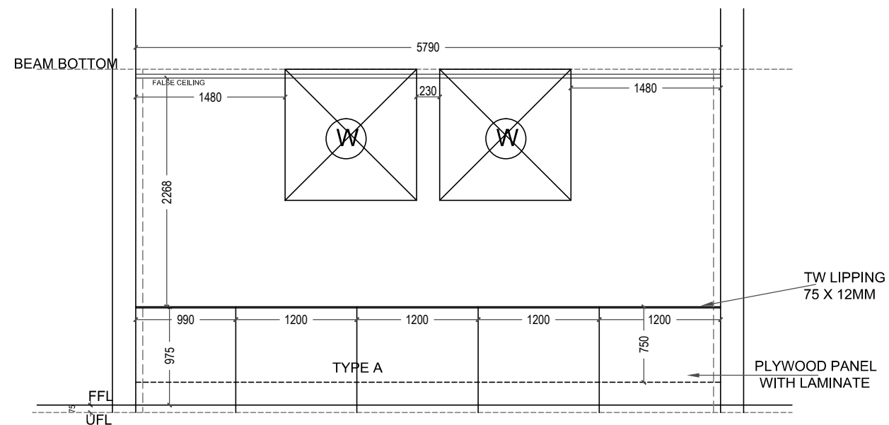
ELEVATION A
