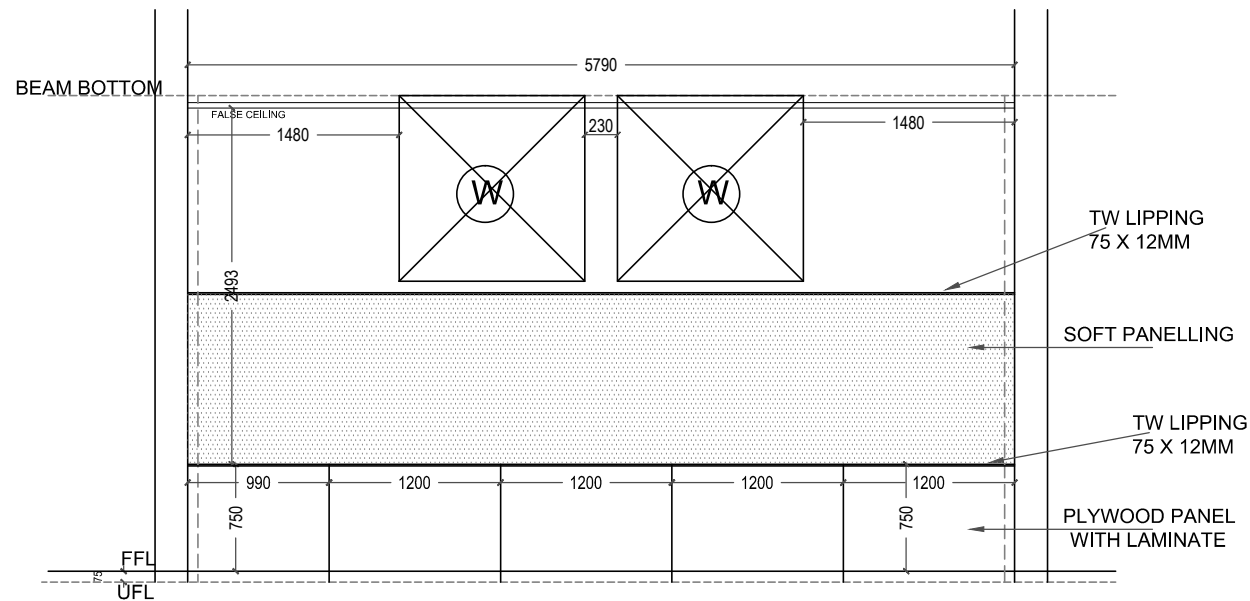
ELEVATION A
